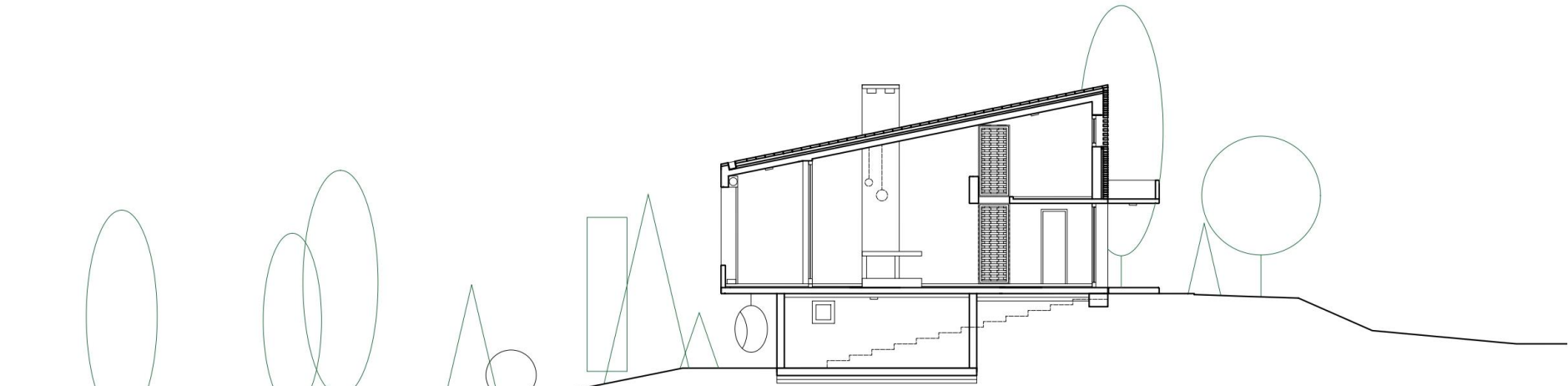
0 1 2 3m LONGITUDINAL SECTION
