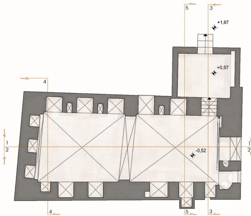
Figure 6 Scale: 1:200
