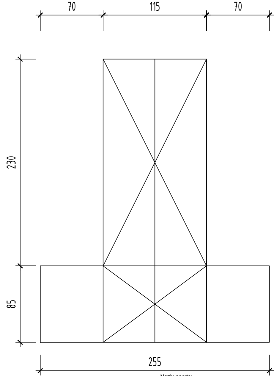
Naziv nacrt: DETALJ obloge prozora od perforiranog MDF-a M2
