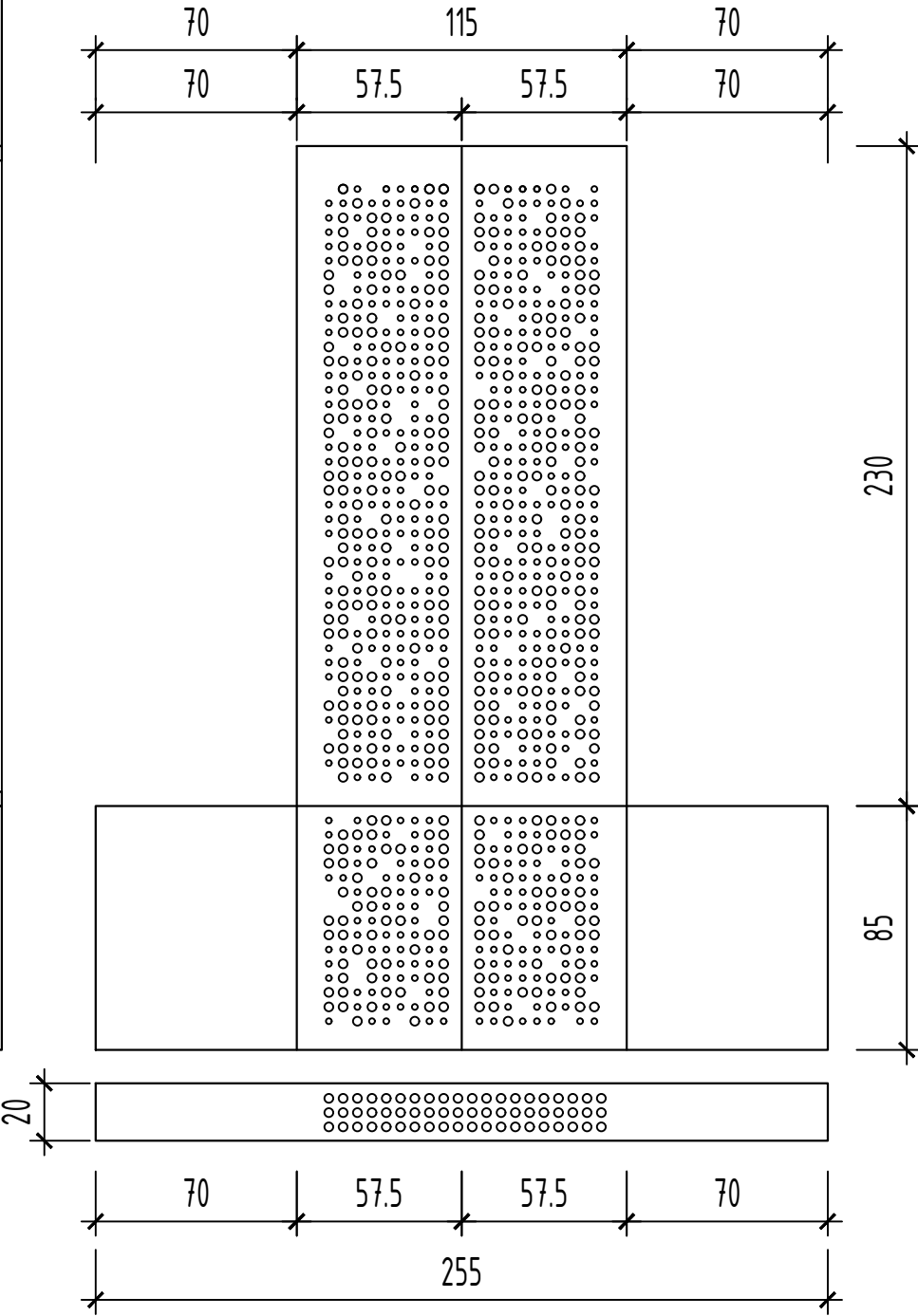
Naziv nacrt: DETALJ obloge prozora od perforiranog MDF-a M2 zlatna boja Capadecor CapaGold
