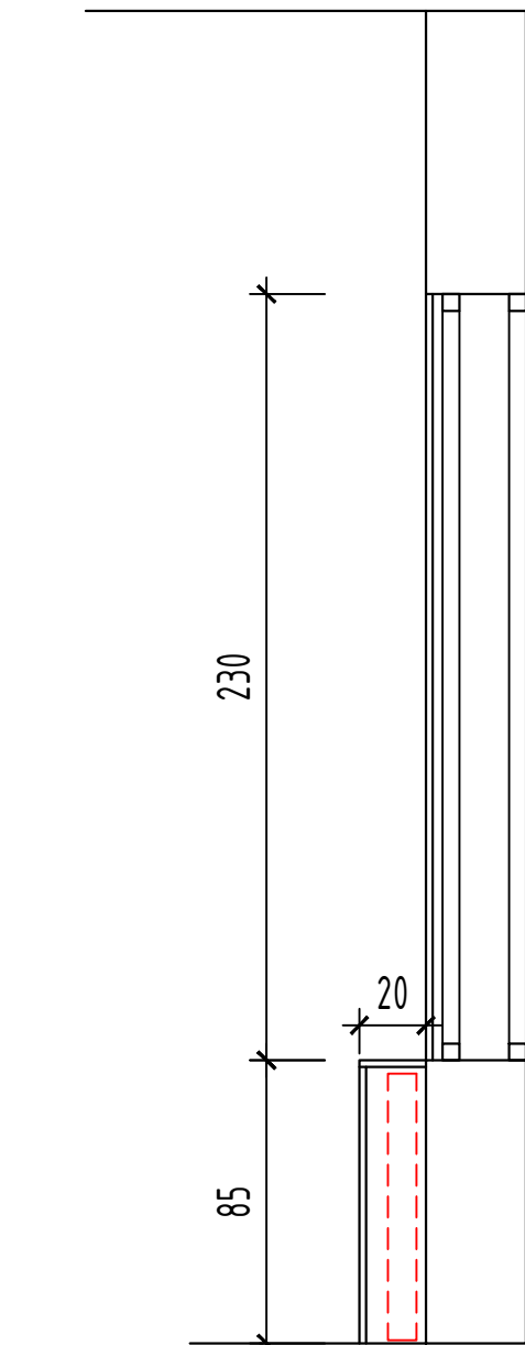
Naziv nacrt: DETALJ obloge prozora od perforiranog MDF-a M2 zlatna boja Capadecor CapaGold
