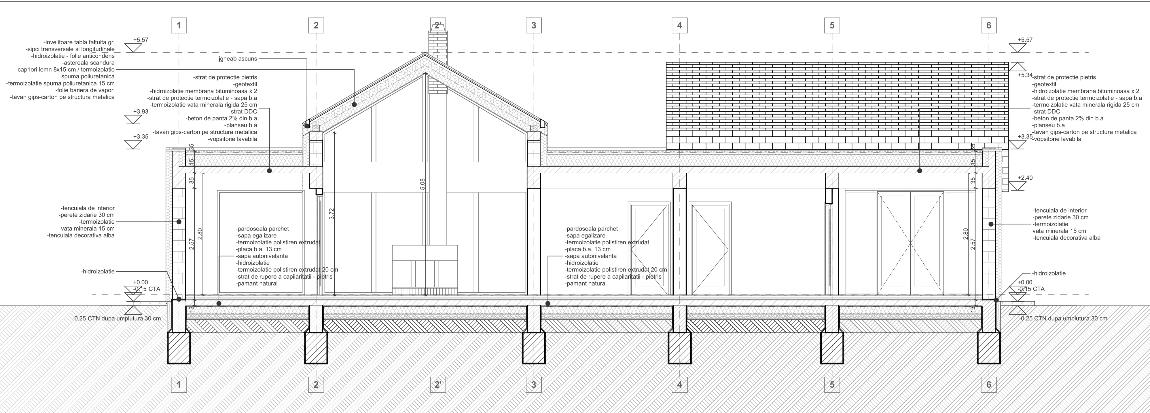
Sectiune longitudinala A-A 1
